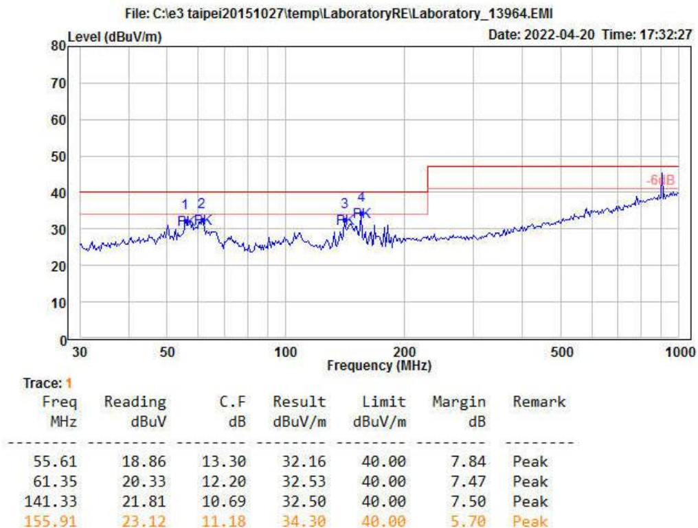
图 5-7 辐射测试垂直方向
