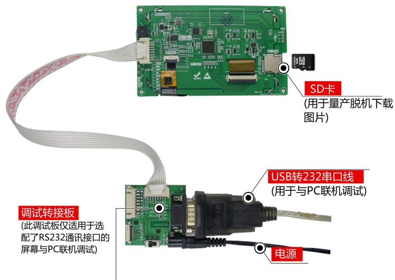
图 1-5 调试工具图
