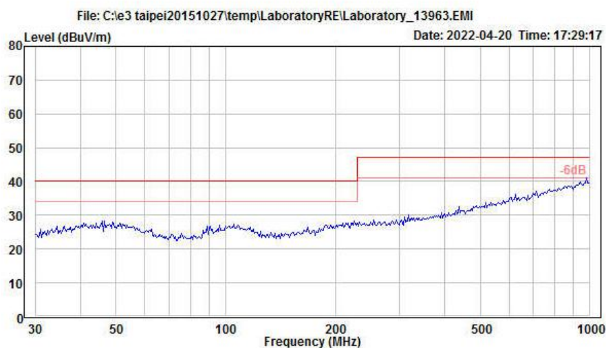
图 5-6 辐射测试水平方向
