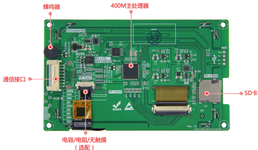
图 1-4 硬件配置图
